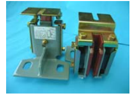
mitsubishi GUIDE SHOE 8K ร่อง 10 มม.
