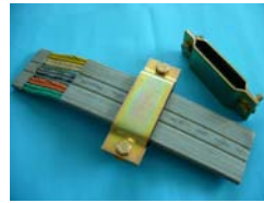
FLAT CABLE CLAMP เหล็กประกบกับเบิ้ลแบน
